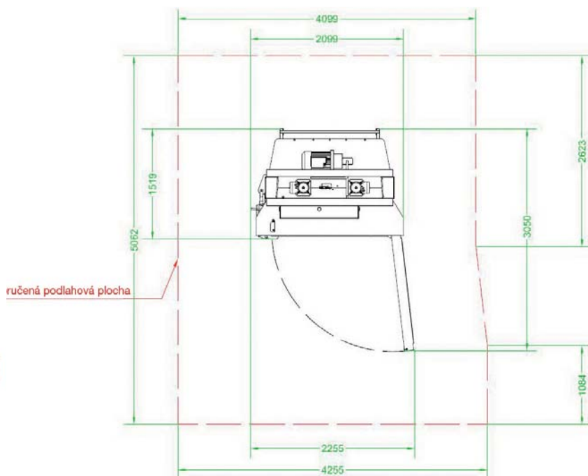
PŮDORYS STROJE
