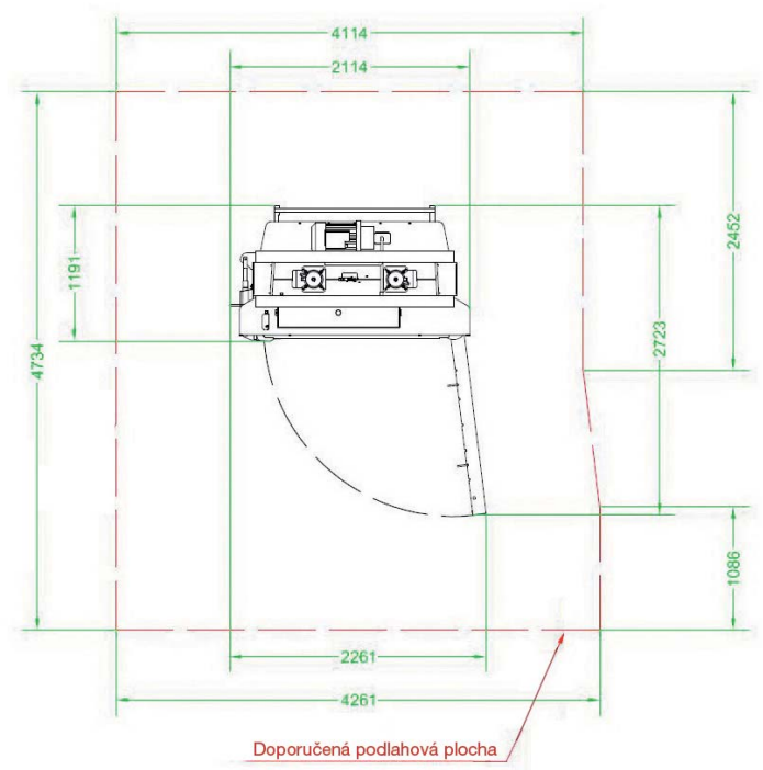
PŮDORYS STROJE
