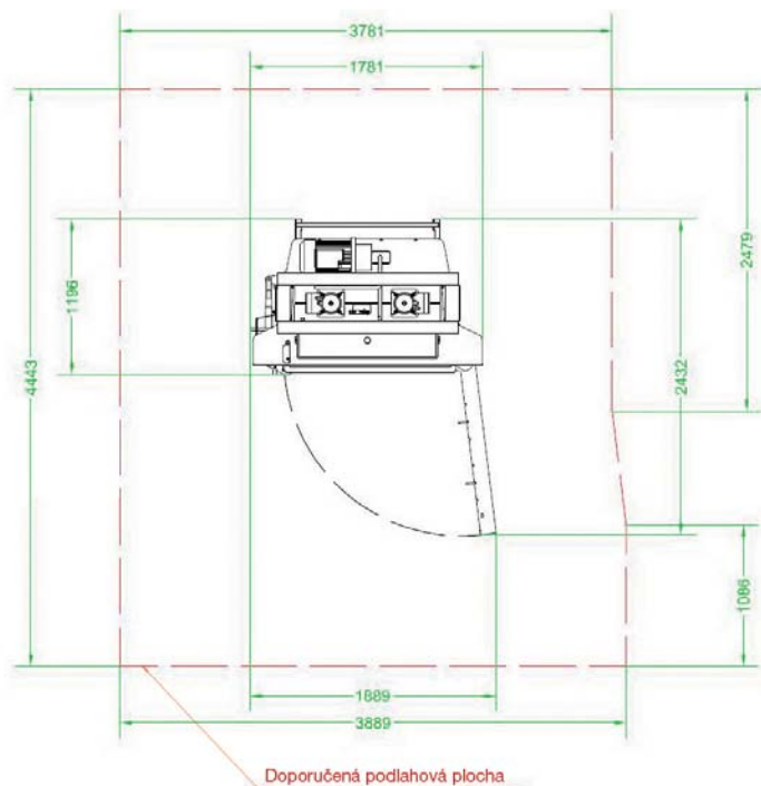
PŮDORYS STROJE
