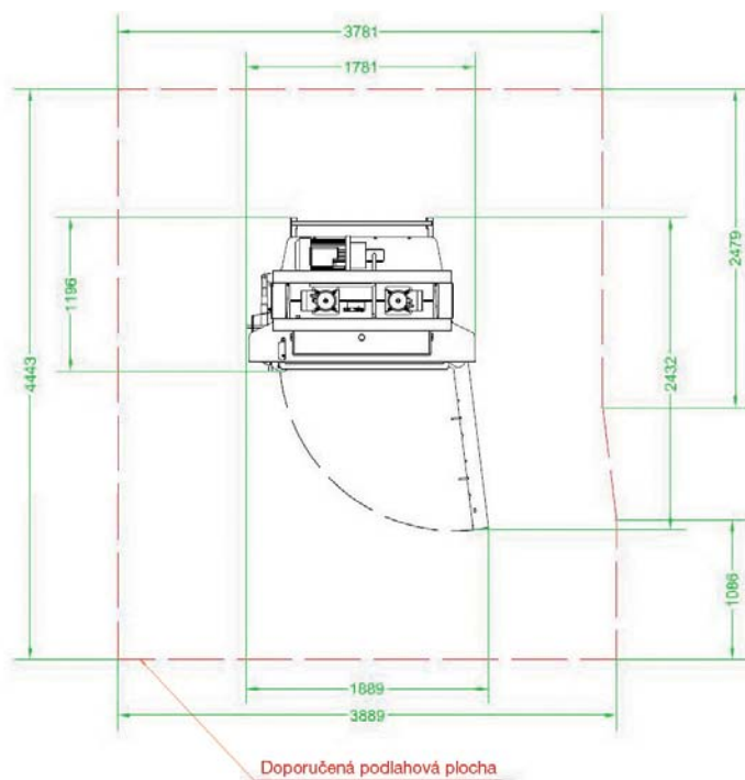
PŮDORYS STROJE
