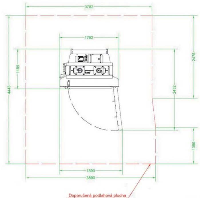
PŮDORYS STROJE
