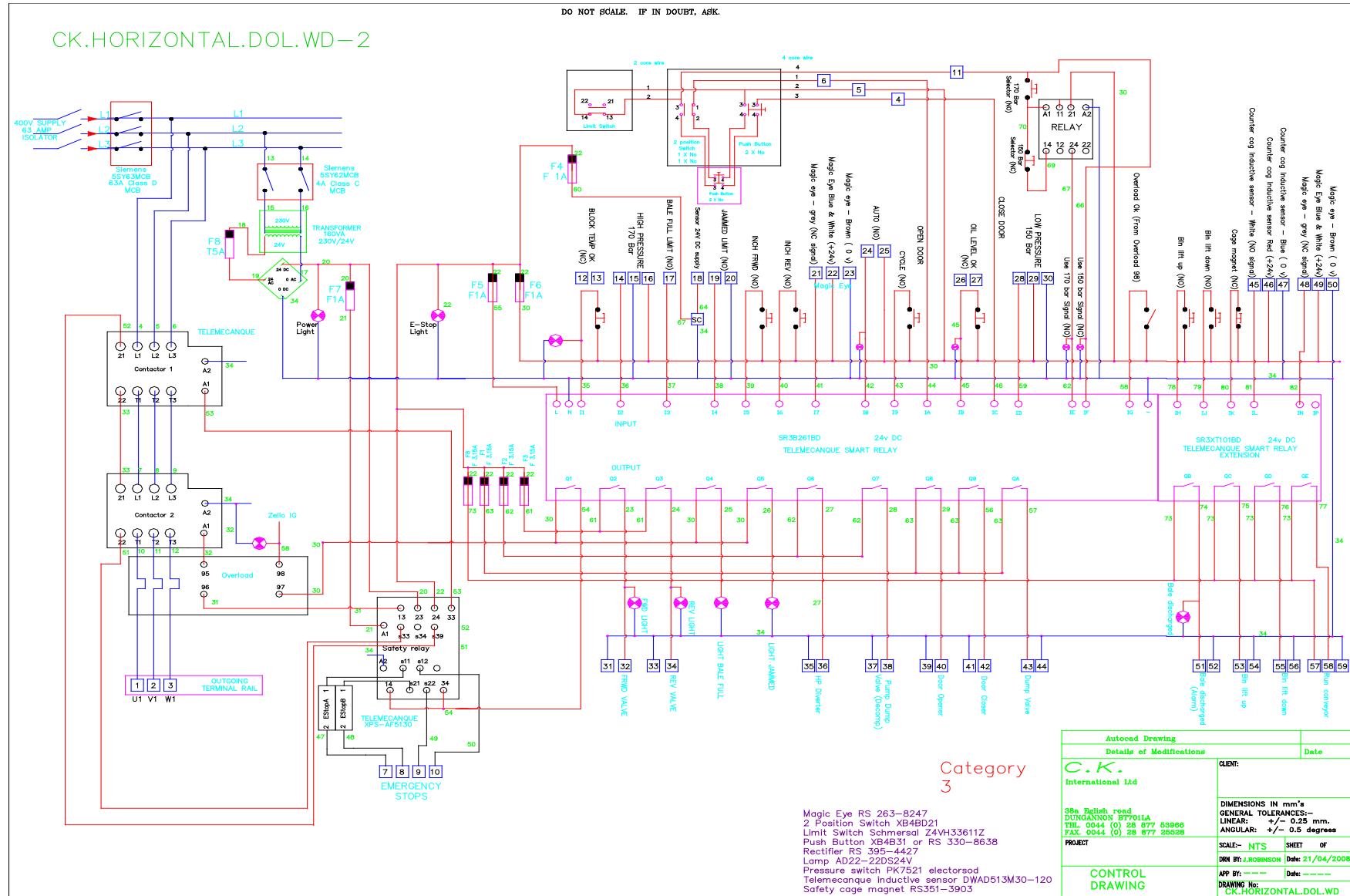
Obr. 2. Elektrické schéma
